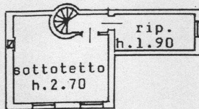
PIANTA SOTTOTETTO
