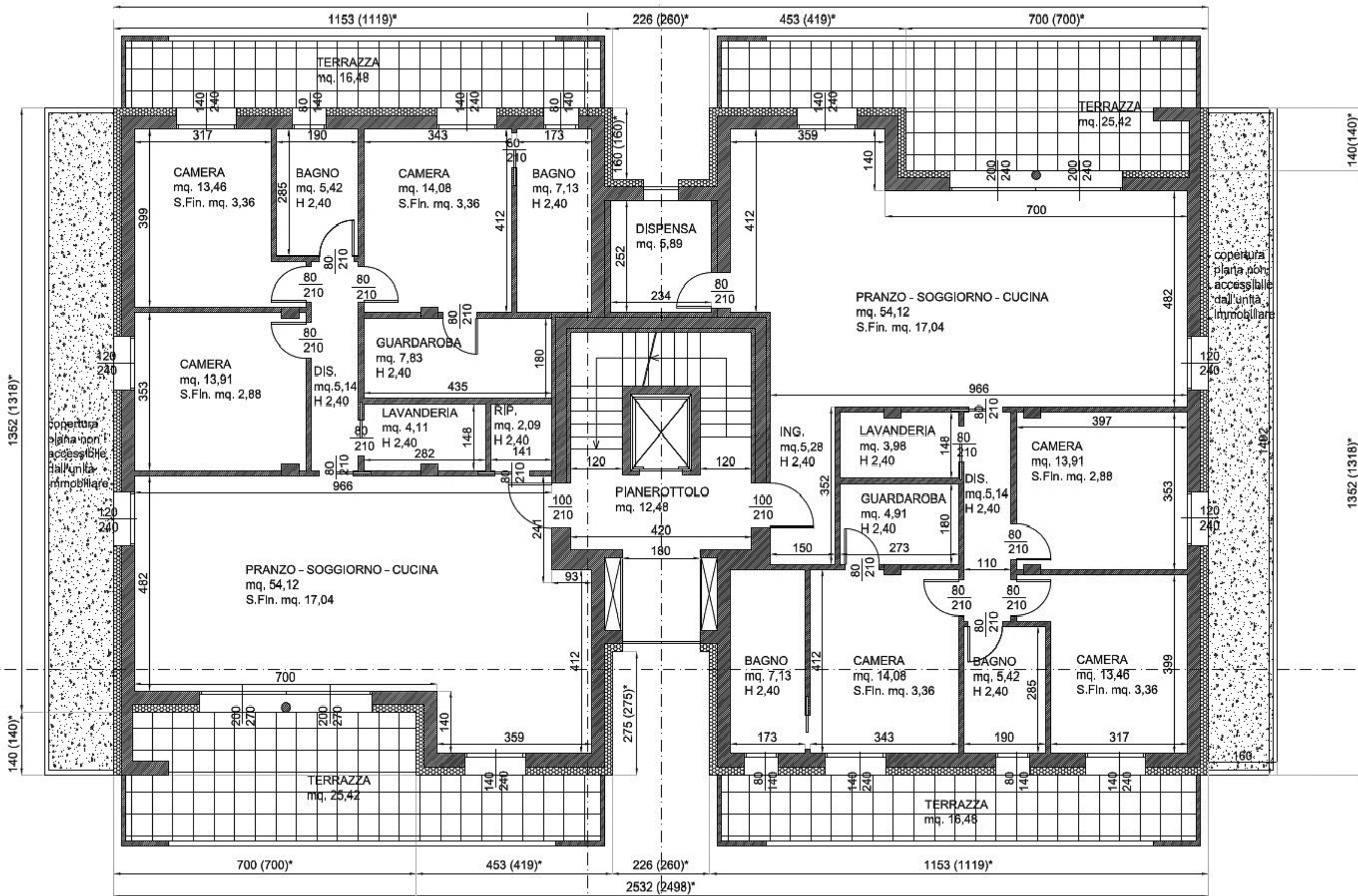
PIANO PRIMO sc. 1:100
