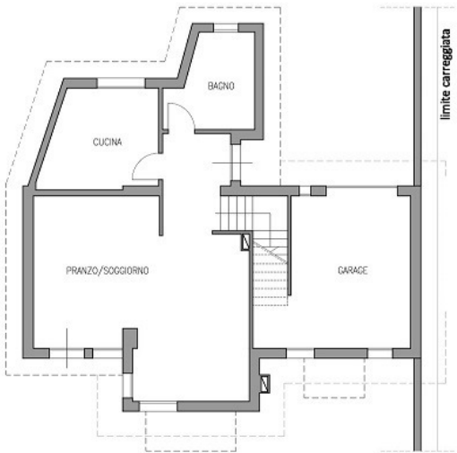
PIANTA PIANO TERRA SCALA 1:100
